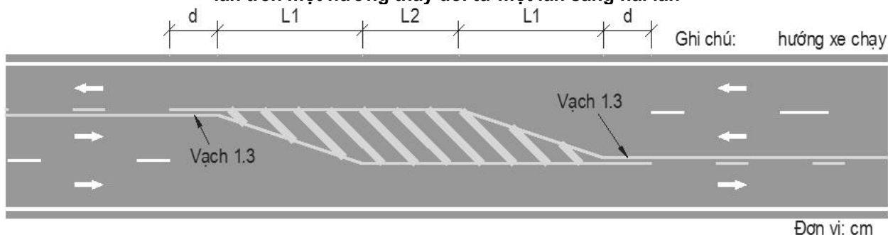
Hình G.9 - Bố trí vạch sơn phân chia hai chiều xe chạy cho đường có 3 làn xe trong khu vực số làn trên một hướng thay đổi từ hai làn sang một làn
