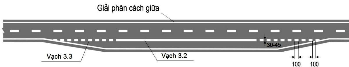
Hình G.18 - Bố trí vạch ở điểm dừng xe kiểu bến cảng không có đảo sơn phân làn
